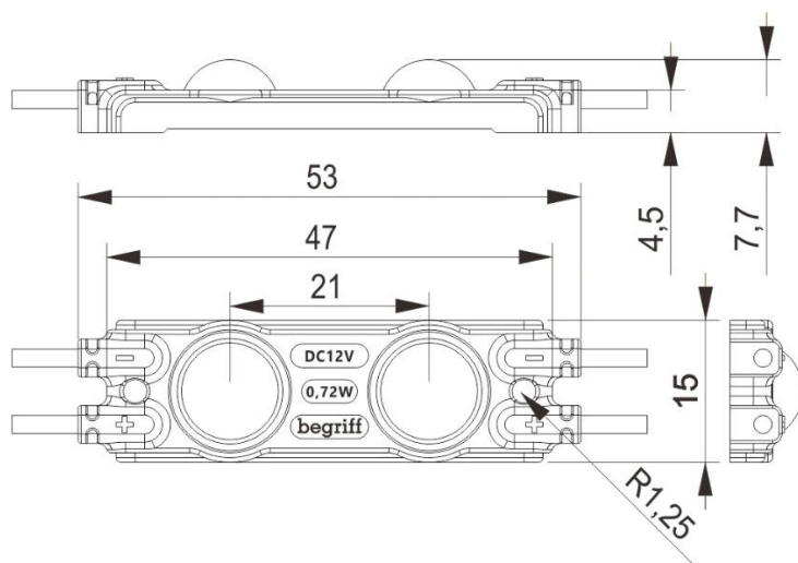
Рис. 2 Размеры модуля
